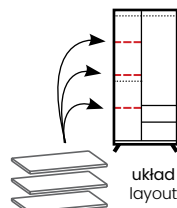
AT 12 - półki do szafy AT11 (3szt) → / ↗ / ↑ 39/48/1,6
