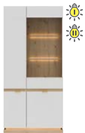
ML 07 - szafka L/P → / × / ↑ 54,5 / 40,5 / 193,5
