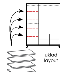
AT 14 - półki do szafy AT13 (4szt) → / ↗ / ↑ 57/48/1,6
